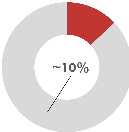
H-Acid
